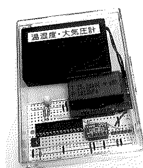
製作された 電子温湿度・大気圧計
